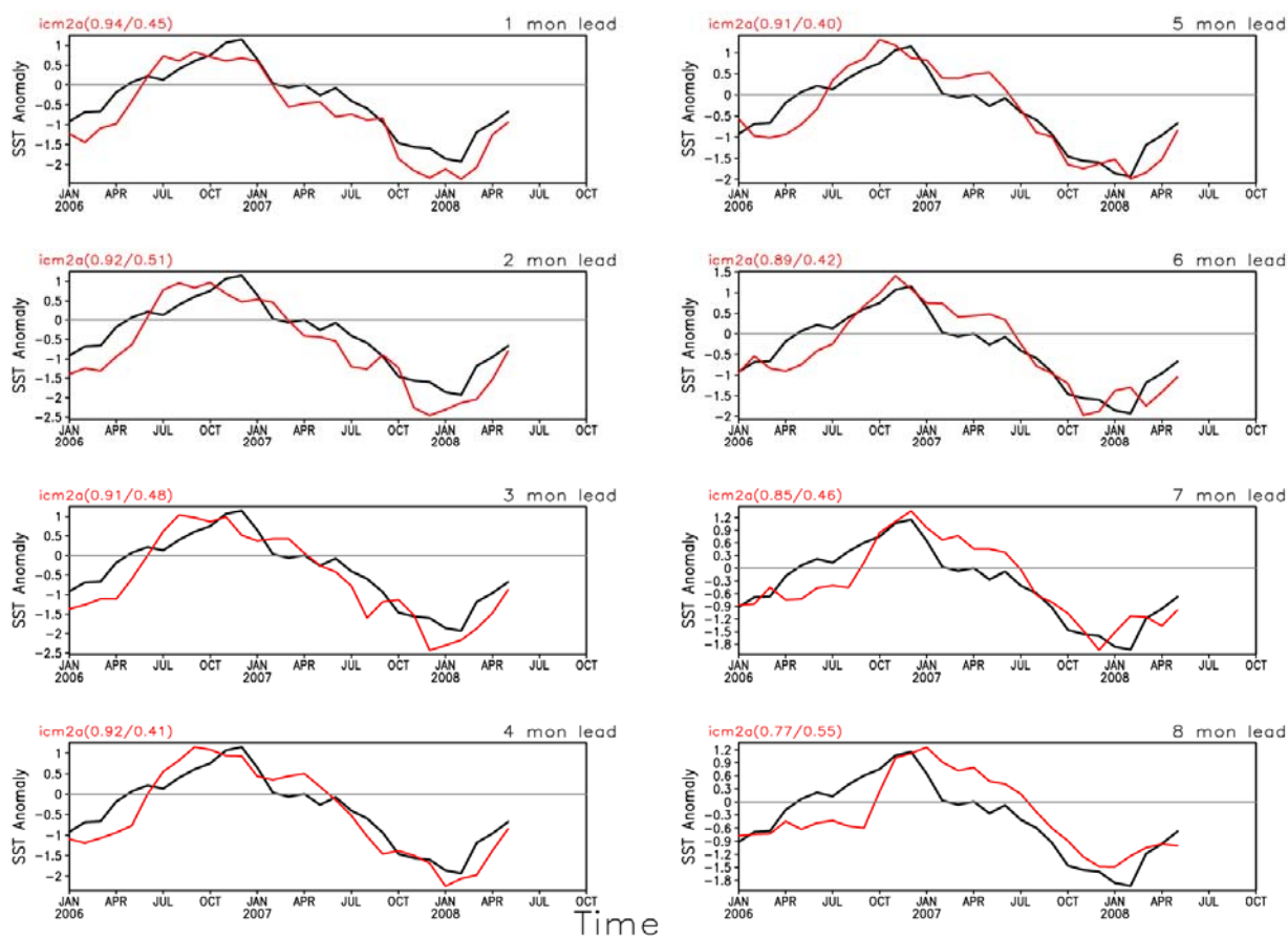
圖 7. 如圖 3 但為 ICM2a 模式，由上而下，由左而右分別為 lead1-lead8 (紅線)，黑線為觀測海溫。
