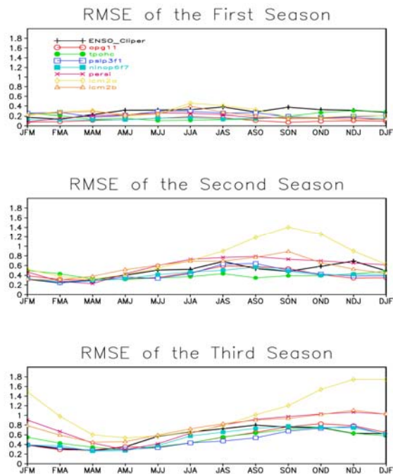
圖 2. 各個模式(不同顏色的線)和 ENSO Cliper(黑線)對 NINO3.4 區海溫的 root mean square error.。橫軸為所預報的季節;直軸為 root mean square
