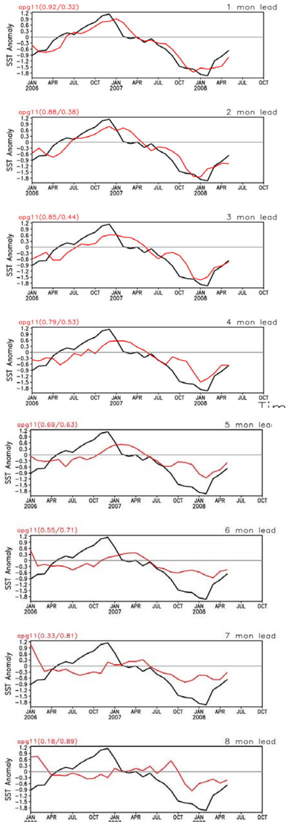
圖 3. OPGSST 模式 lead1 至 lead8 (由上至下) 之預
