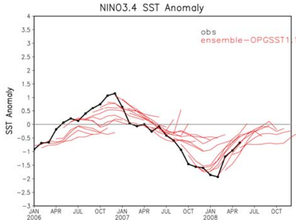
圖 4. OPGSST 模式作業性預報（西元 2006 年 1 月至 2008 年 5 月）（細線）與觀測資料（實線）對 NINO3.4 的平均海溫。細線為 OPGSST 模式每個月預報。
