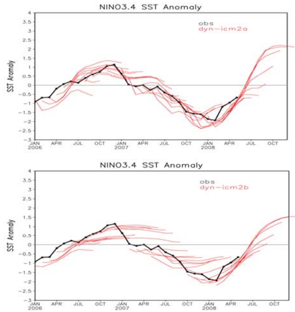
圖 6. 如圖 4 但為 2 個動力模式，由上而下，分別為 ICM2a 和 ICM2b。
