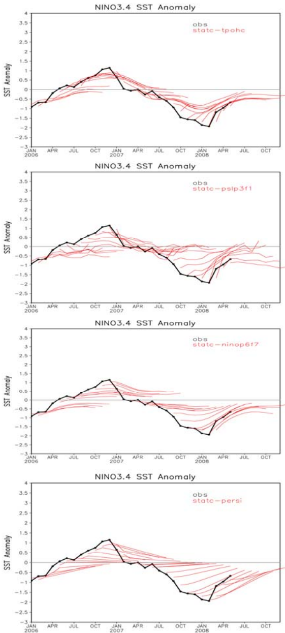
圖 4. OPGSST 模式作業性預報（西元 2006 年 1 月至 2008 年 5 月）（細線）與觀測資料（實線）對 NINO3.4 的平均海溫。細線為 OPGSST 模式每個月預報。
