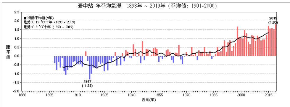
圖3，同圖2，但為1898-2019年臺中測站之溫度距平時序圖。
