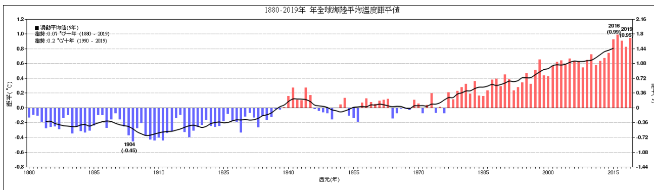
圖1. 1880-2019年全球溫度距平之時間序列圖，圖中紅色/藍色長條分別表示正距平/負距平溫度，5年滑動平均為黑色實線，圖左上數值分別為百年及>近30年之上升趨勢值，單位為°C/10年。
