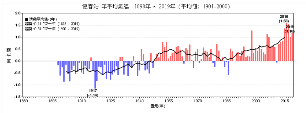
圖6，同圖2，但為1898-2019年恆春測站之溫度距平時間序列圖。
