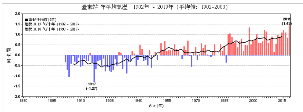
圖8，同圖2，但為1902-2019年臺東測站之溫度距平時間序列圖。
