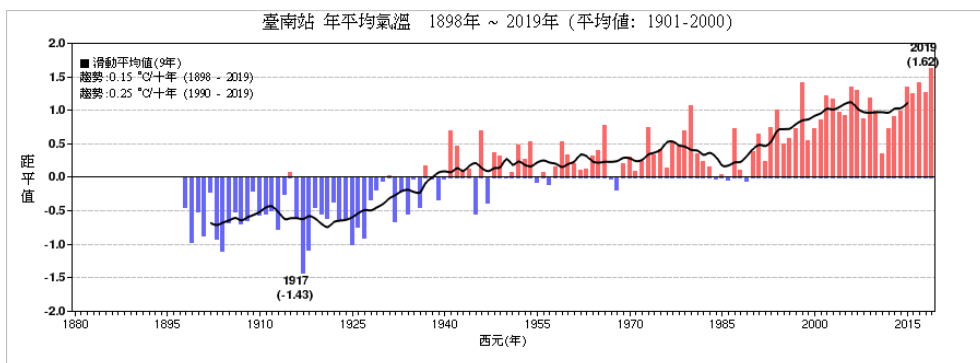
圖4，同圖2，但為1898-2019年臺南測站之溫度距平時序圖。
