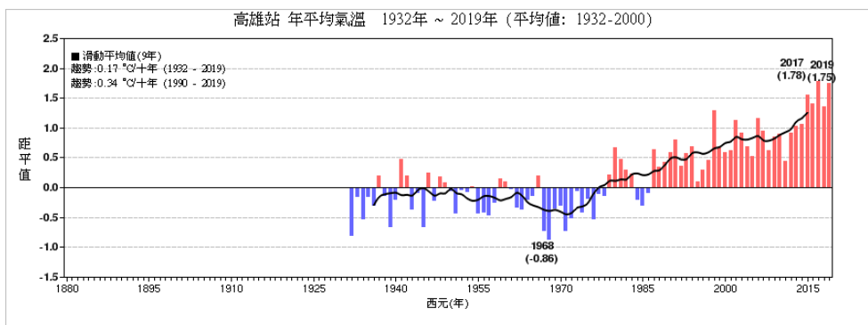
圖5，同圖2，但為1932-2019年高雄測站之溫度距平時間序列圖。
