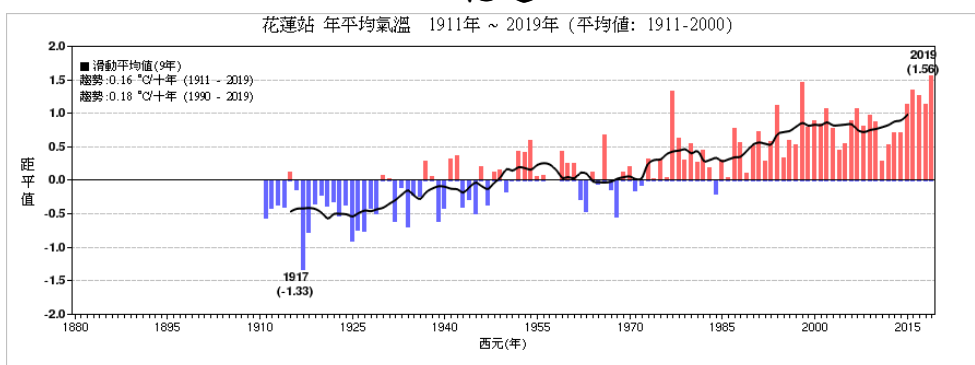
圖7，同圖2，但為1911-2019年花蓮測站之溫度距平時間序列圖。
