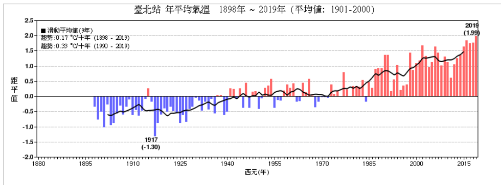
圖2，1898-2019年臺北測站之溫度距平時序圖，圖中紅色/藍色長條分別表示正距平/負距平溫度、5日滑動平均（黑實線）、百年迴歸趨勢線（紅虛線）及近30年迴歸趨勢線（綠虛線），單位為 ^{\circ}\text{C} ，圖中左上方數值分別為百年及近30年之上升趨勢值，單位為 ^{\circ}\text{C}/10 年
